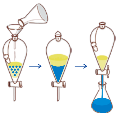
《図2 分液漏斗による油性成分の水洗作業》
